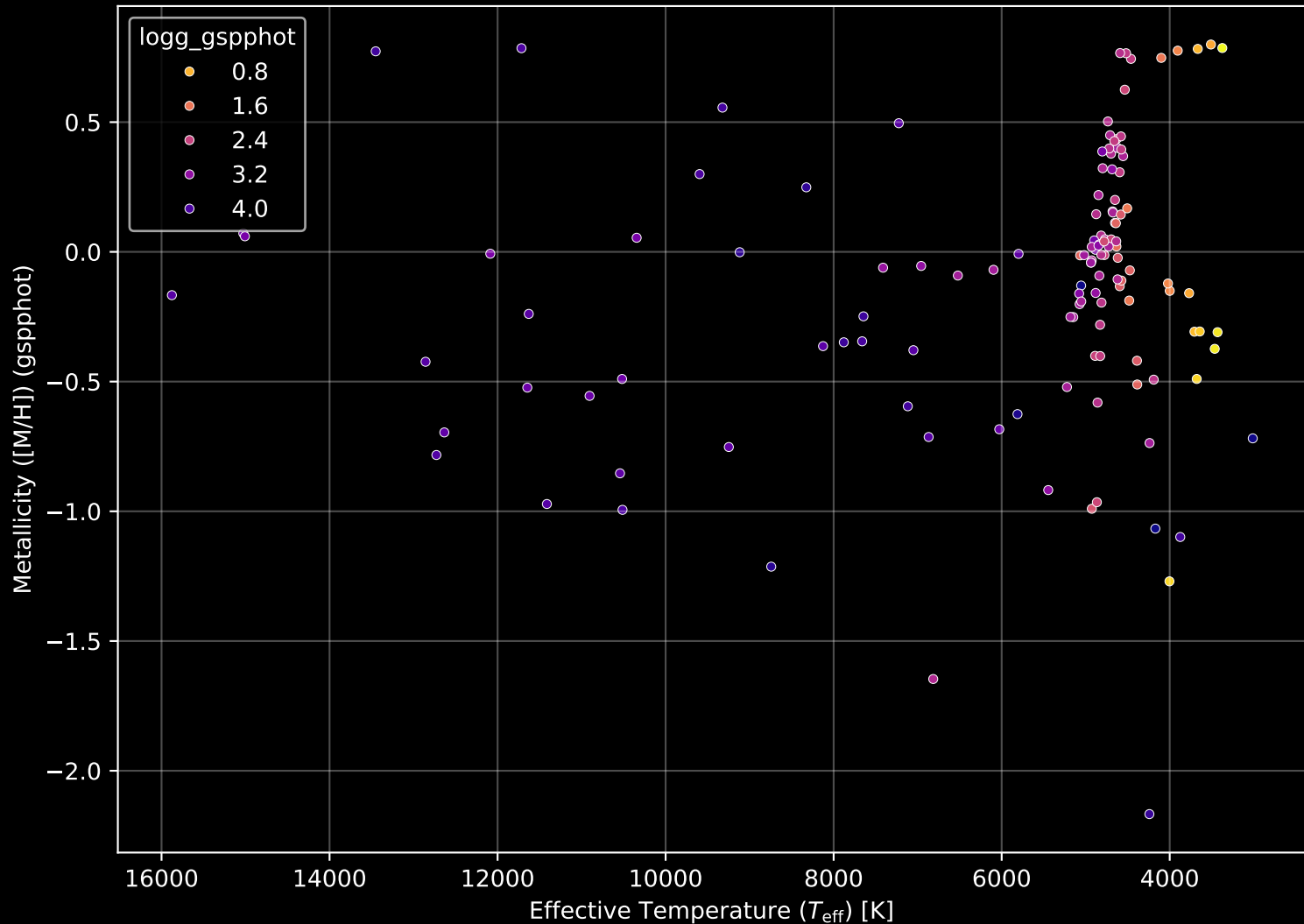
APOGEE DR17 Field: [045+00] Stellar Population Parameters (n= 130)
